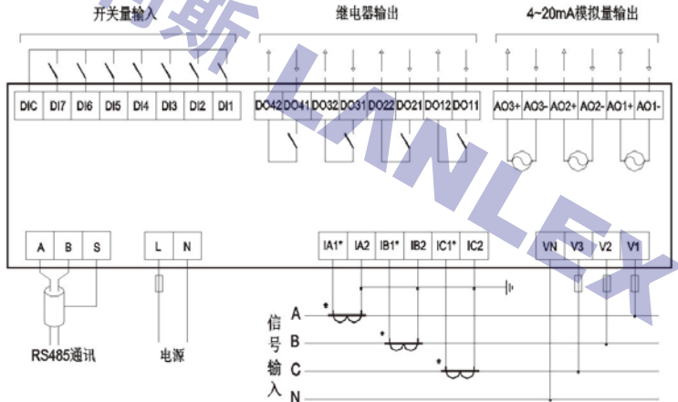
图 4.1.a 装置典型功能接线示意图
