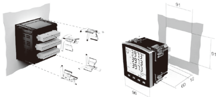
图 7.1.a LS830E/LS930E-9 开孔尺寸及安装方法
