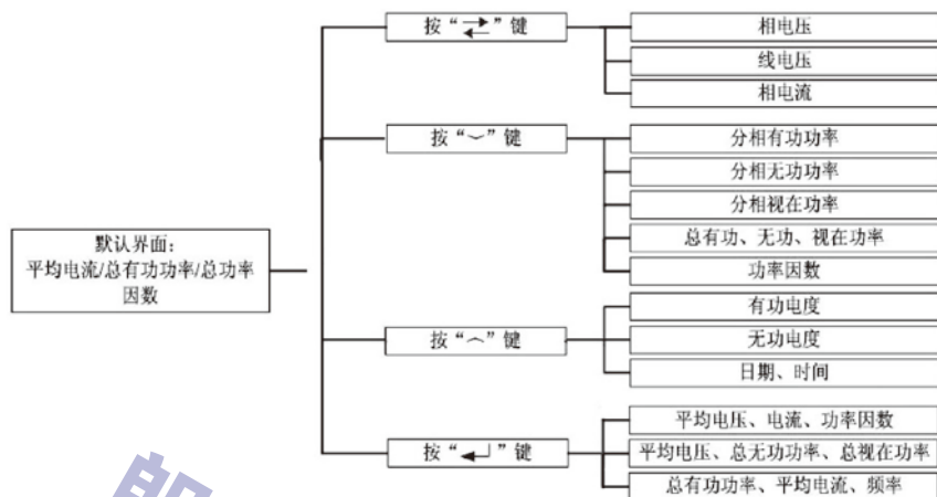
图 5.4.b 液晶装置显示模式菜单总览
